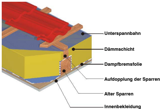
Schnitt durch ein Dach mit einer Dampfbremssfolie, die von außen um die Sparren herum geführt wurde
